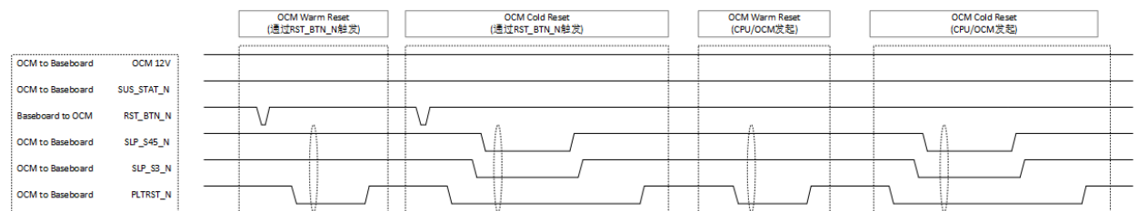
Figure 20 OCM 重启时序
