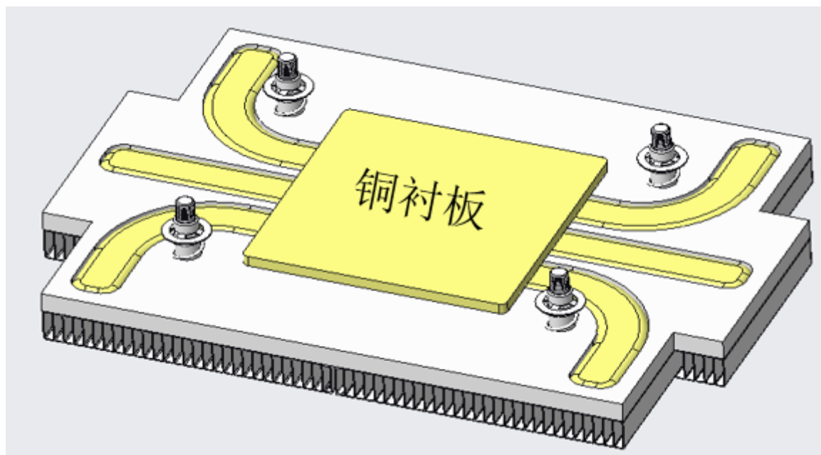
Figure 31 BP-HS 散热器结构
