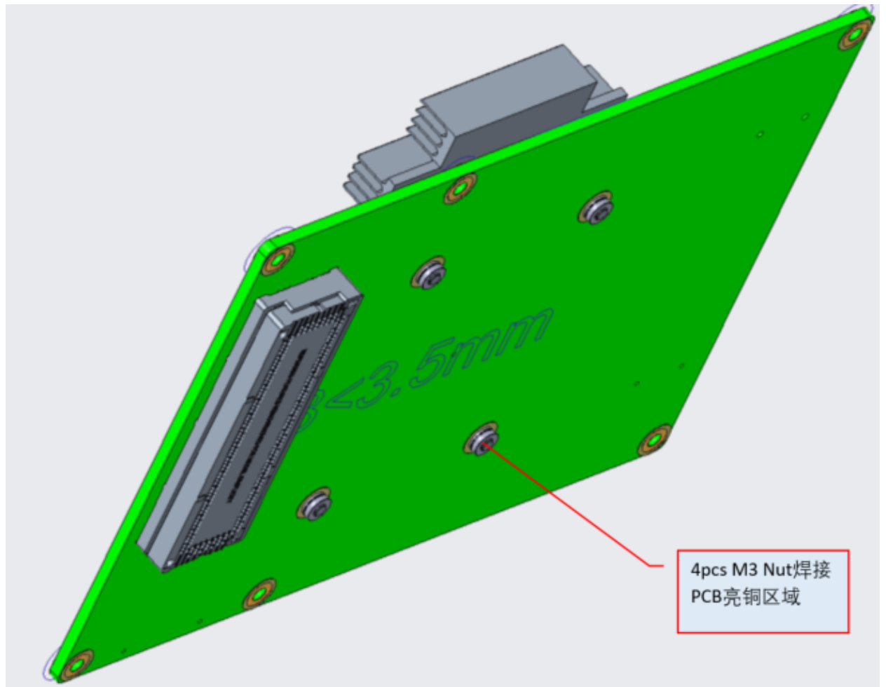
Figure 26 LP-HS 散热器焊接螺母
