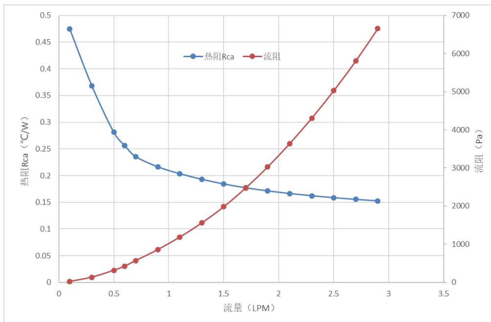
Figure 36 液冷散热器热阻及压差 vs 流量曲线图
