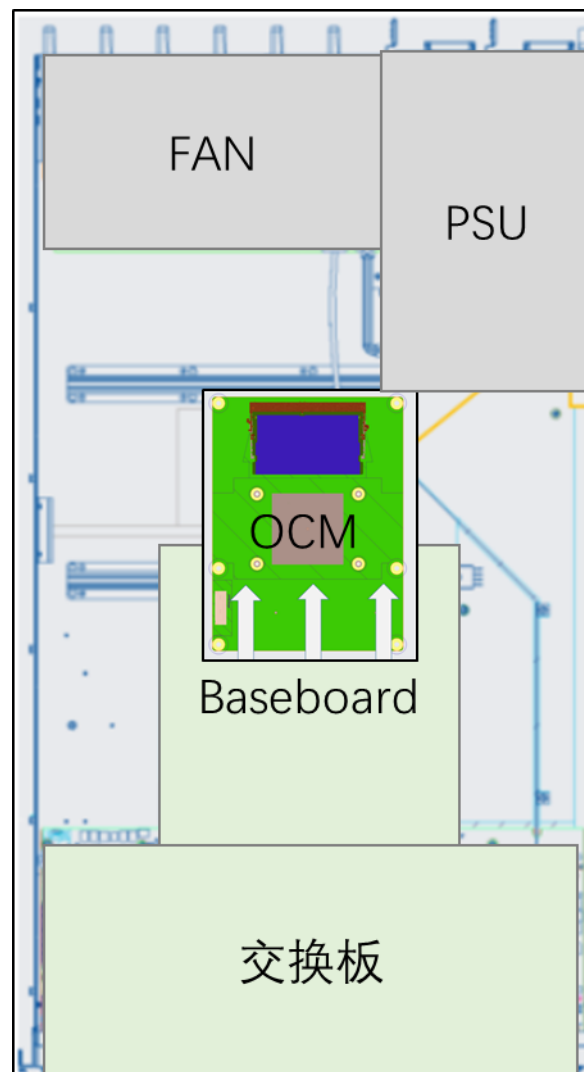
Figure 24 1RU 交换机系统内 OCM 卡组装图
