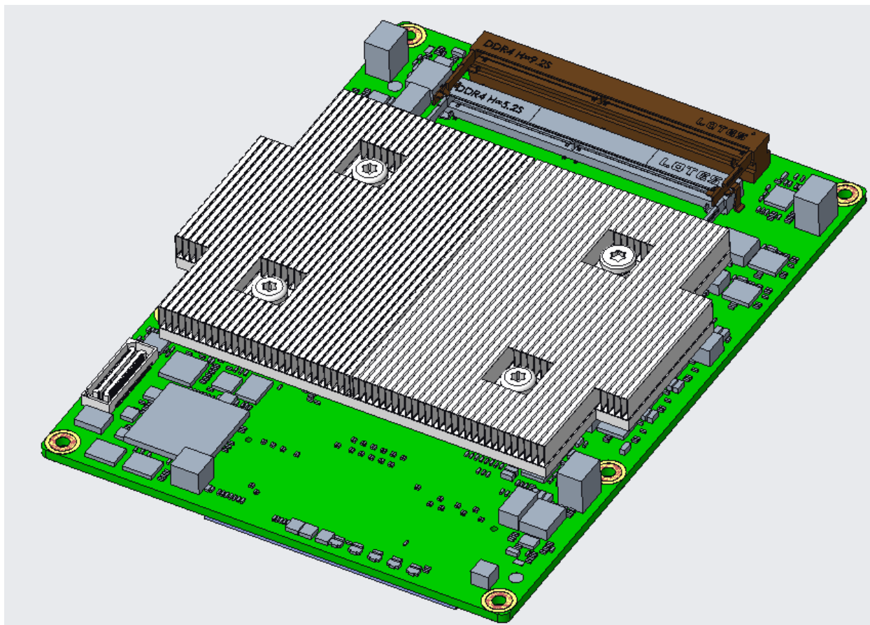
Figure 30 BP-HS 散热器安装图
