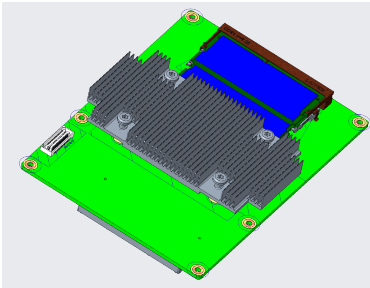
Figure 25 LP-HS 散热器
