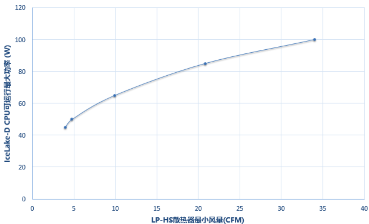
Figure 28 LP-HS 散热器最大可支持 CPU 功耗 Vs 最小风量关系图
