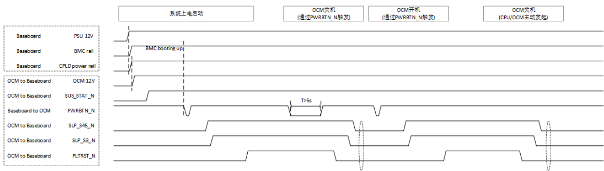
Figure 19 OCM 上下电时序
