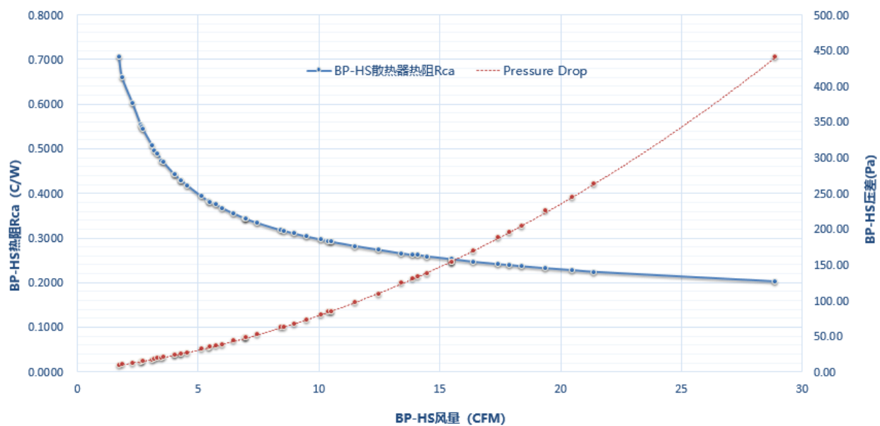
Figure 32 BP-HS 散热器热阻及压差 Vs 风量曲线图
