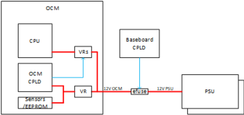
Figure 16 Baseboard 到 OCM 的 12V 供电拓扑
