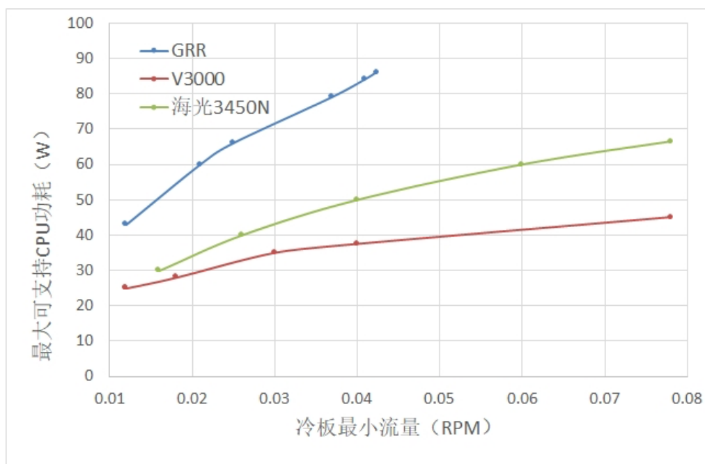
Figure 37 液冷散热器最大可支持 CPU 功耗 Vs 最小流量关系图
