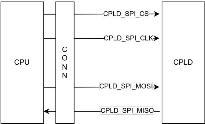
Figure 145 系统 SPI/模拟 SPI 逻辑
