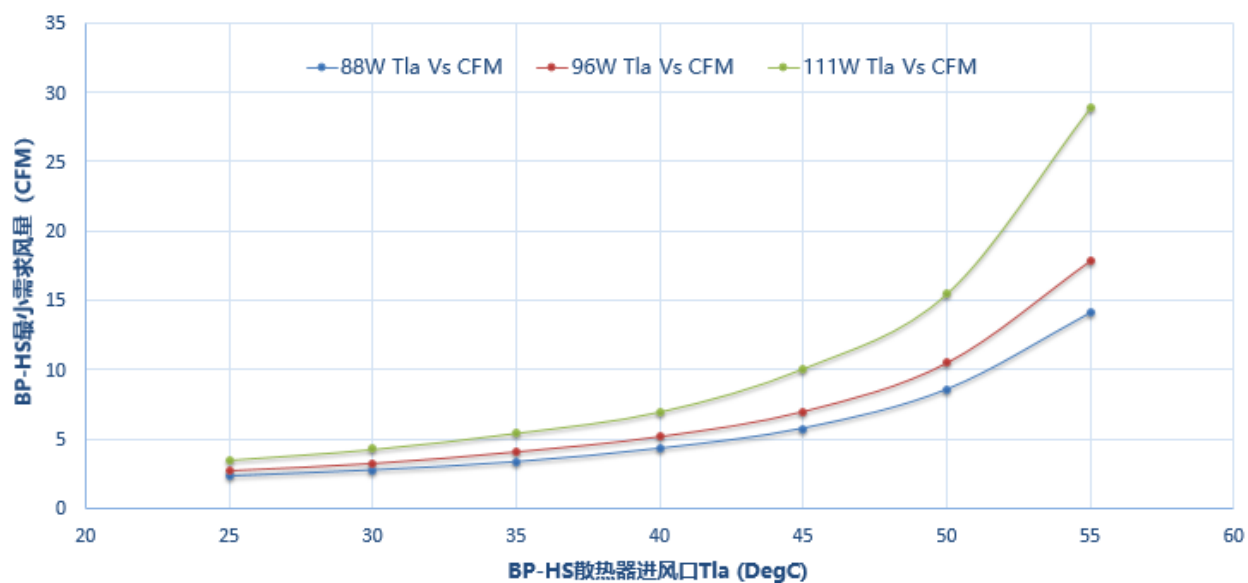
Figure 34 BP-HS 在不同环境温度下所需要最小风量
