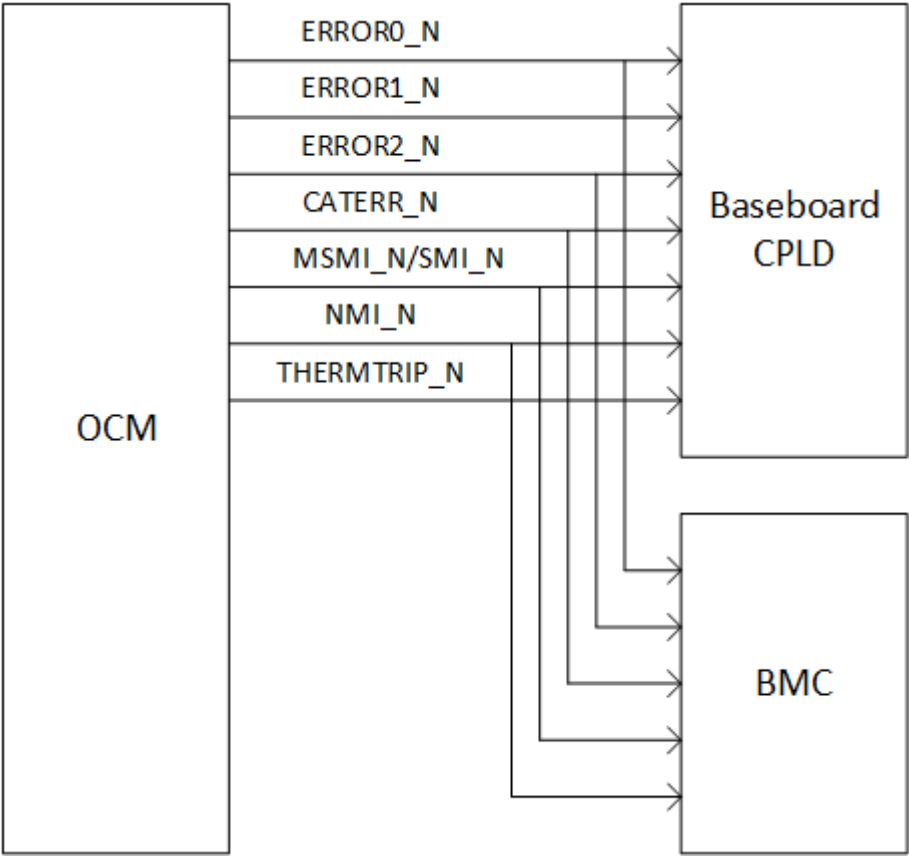
Figure 11 Error 信号处理逻辑
