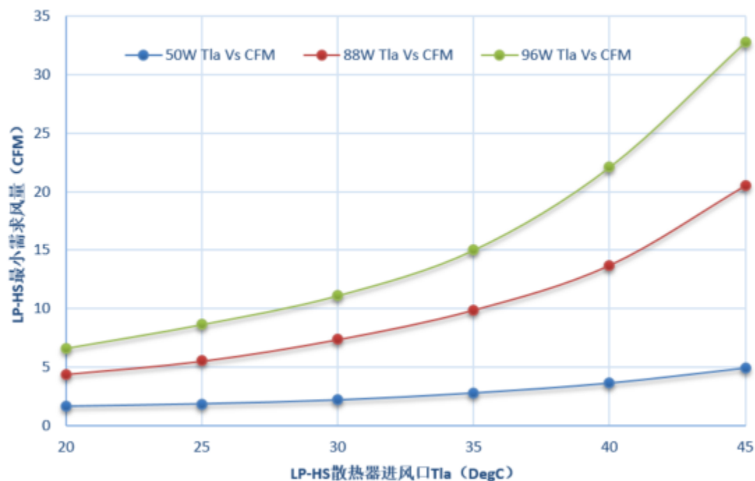
Figure 29 LP-HS 在不同环境温度下所需要最小风量
