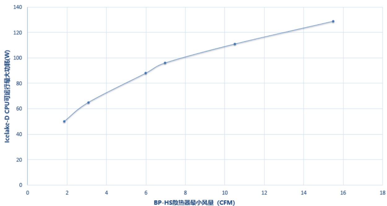
Figure 33 BP-HS 散热器最大可支持 CPU 功耗 Vs 最小风量关系图
