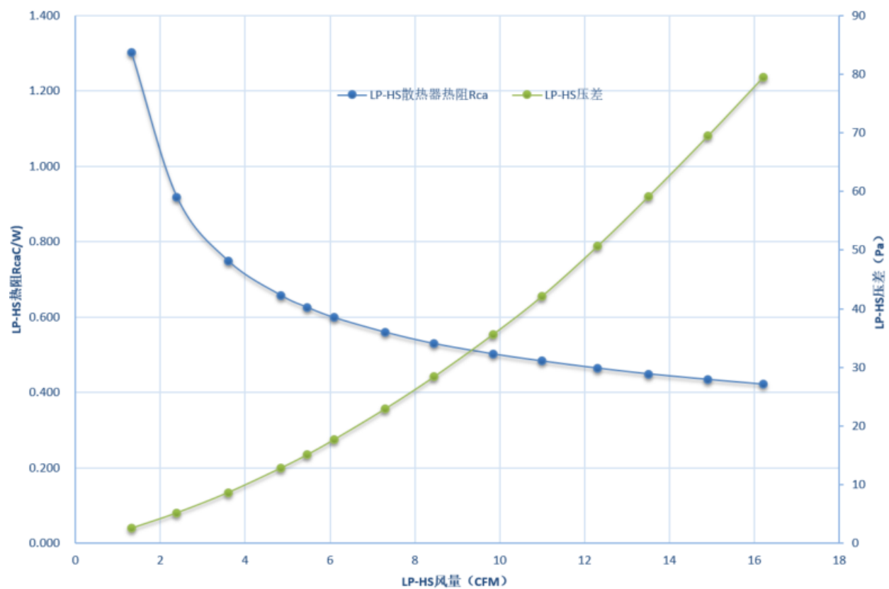
Figure 27 LP-HS 散热器热阻及压差 vs 风量曲线图
