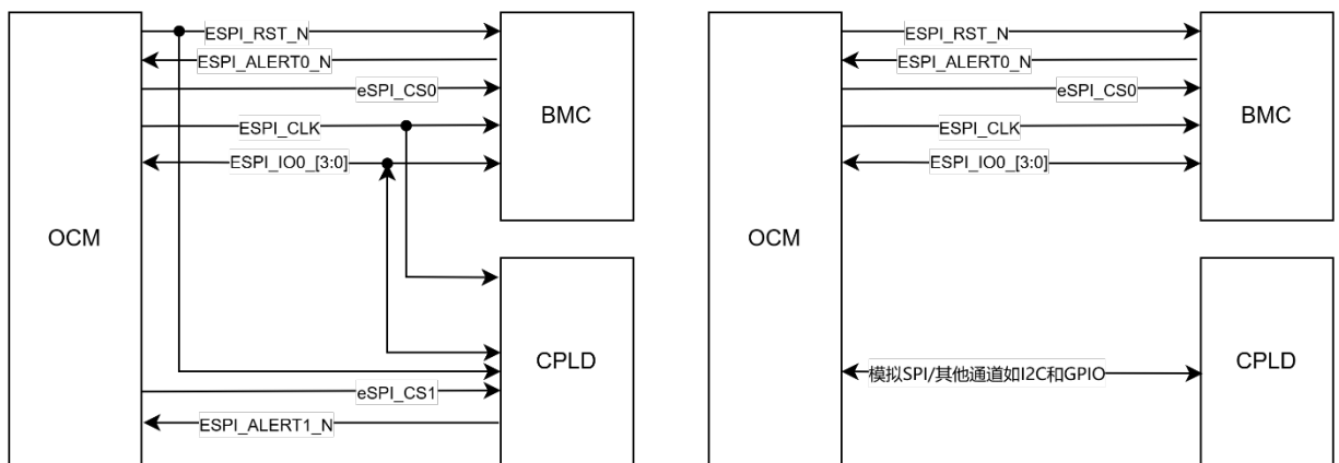
Figure 10 eSPI 场景说明
