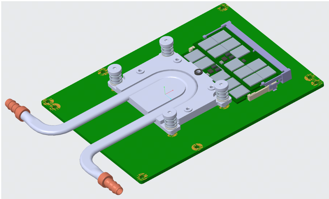
Figure 35 液冷散热器
