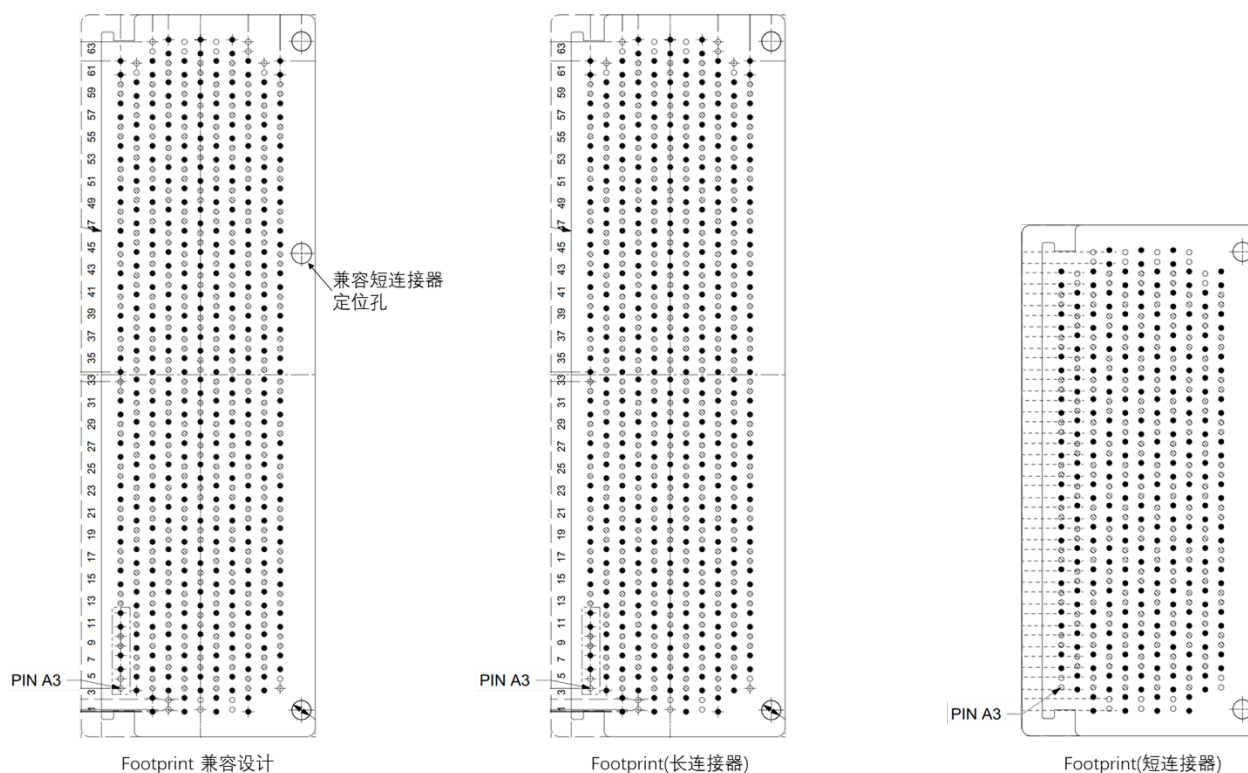
Figure 9 长短连接器兼容设计
