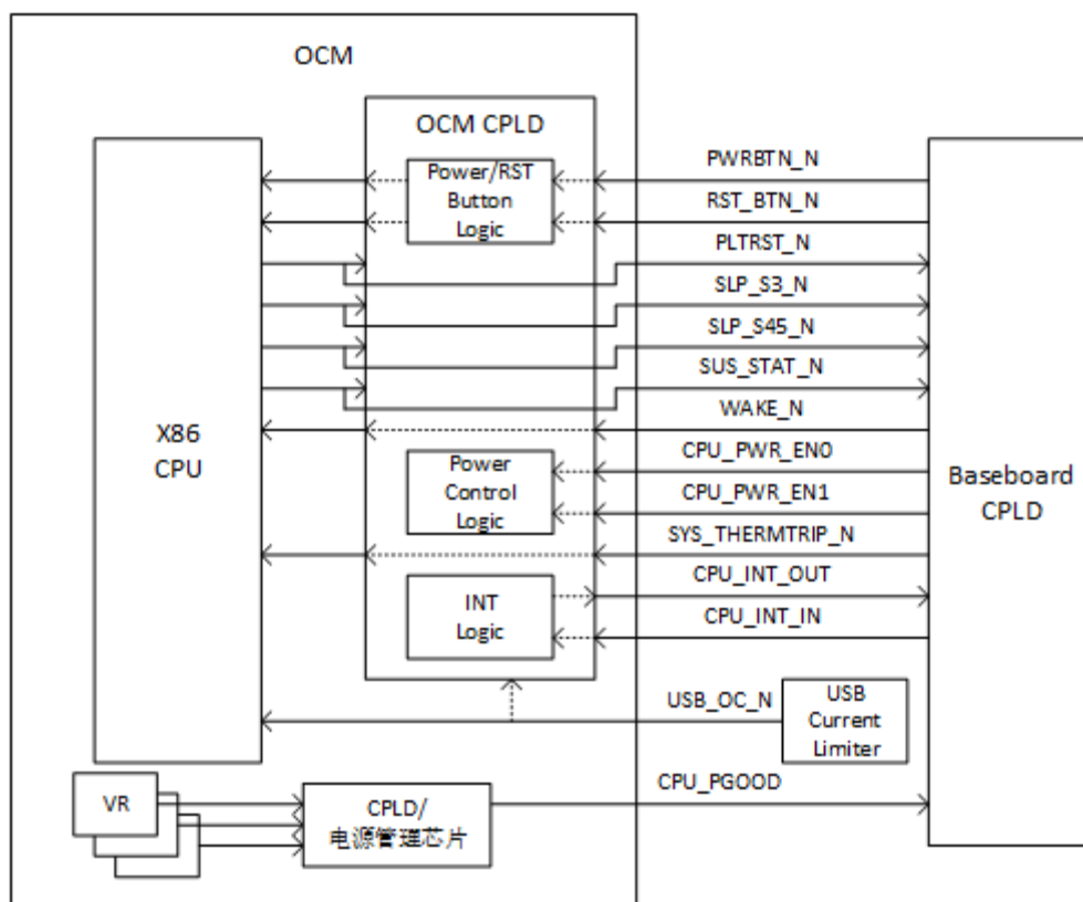
Figure 13 Xeon-D 电源控制、复位处理逻辑
